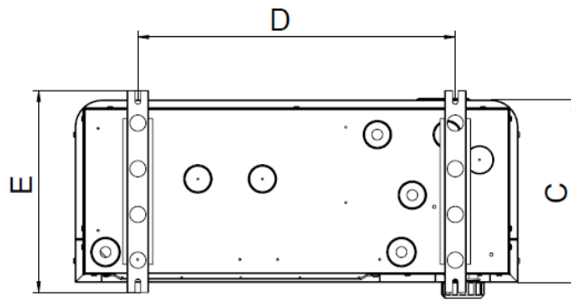
Vorderseite
