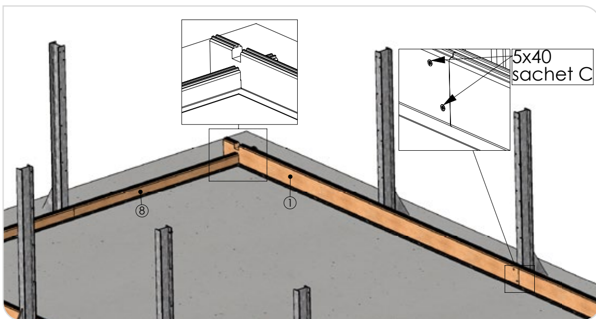
Figure 16 – 1ere rangée de parois
