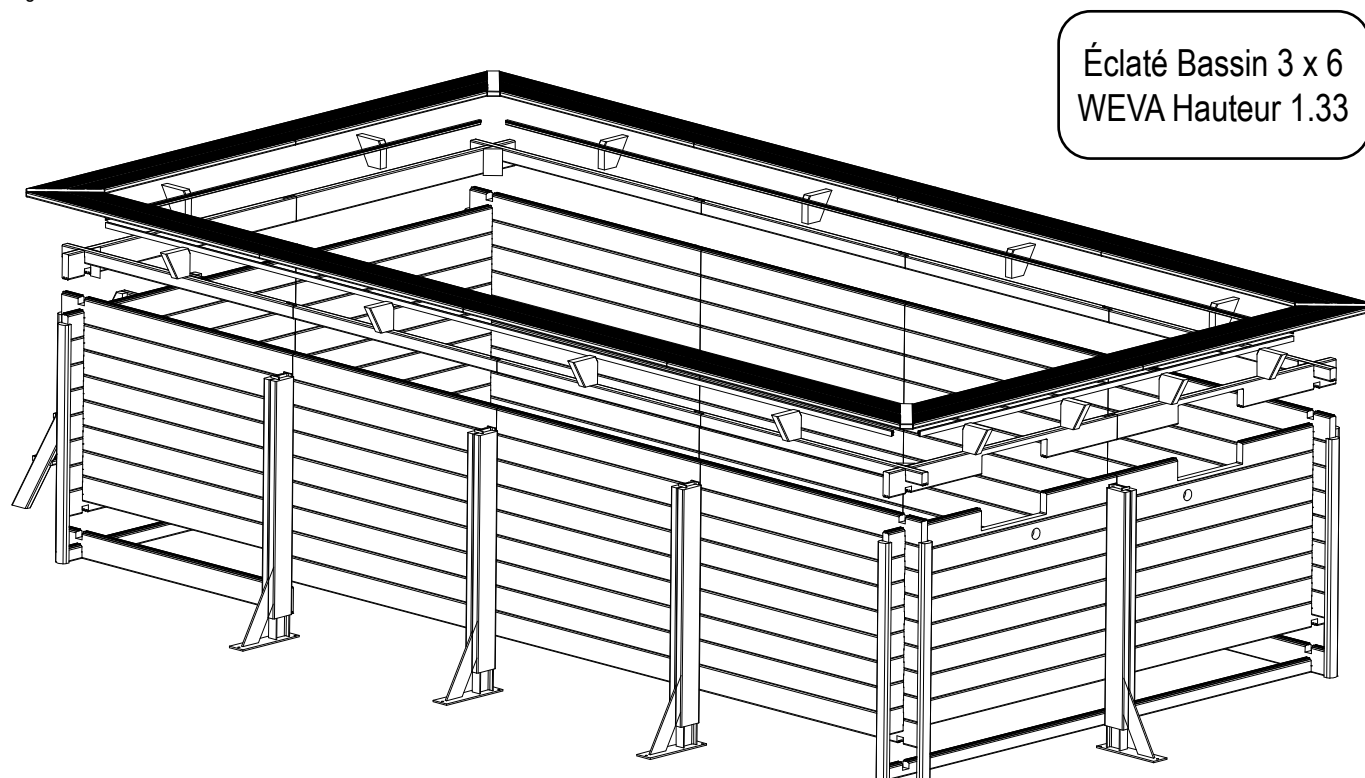
Figure 67 – éclaté bassin 3 x 6 - WEVA hauteur 1.33
