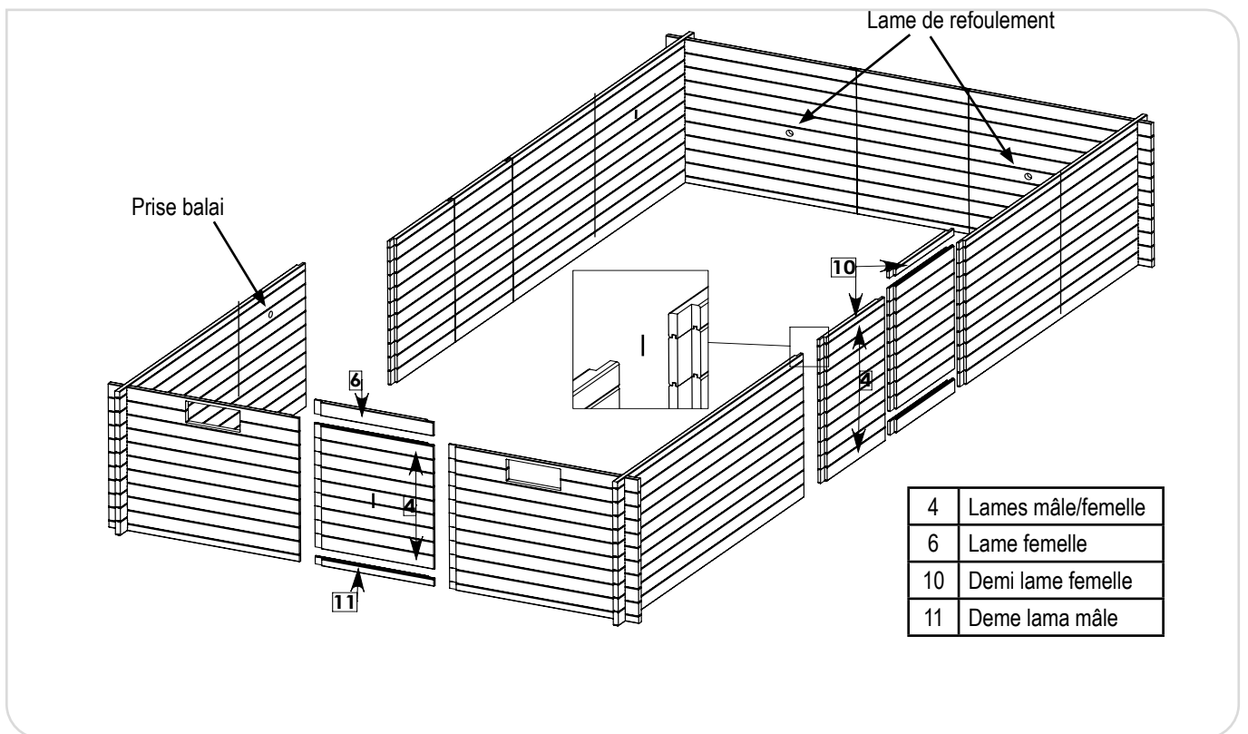
Figure 14 – Emplacement des lames par type - modèle ODYSSEA - 8 x 4
