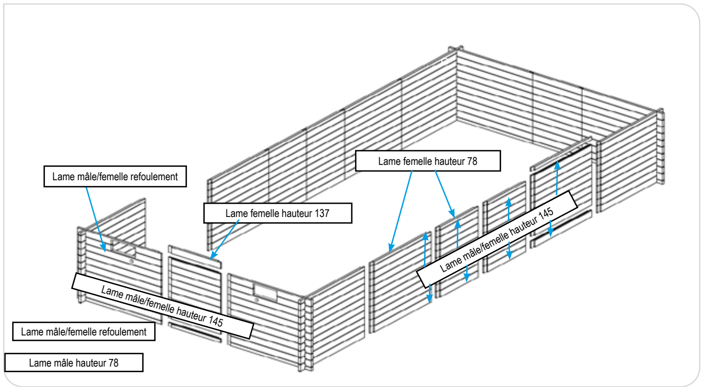
Figure 13 – Emplacement des lames par type - modèle WEVA - 6 x 3
