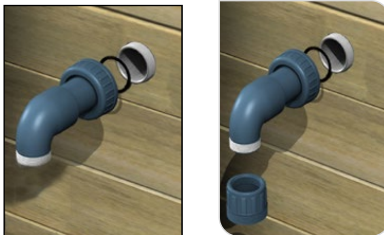
Figure 42 – descente rigide de prise balai - Modèle Odyssea) et Coude sur buses de refoulement
