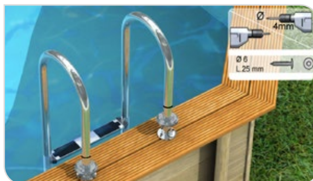
Figure 61 – échelle à l'intérieur de la piscine
