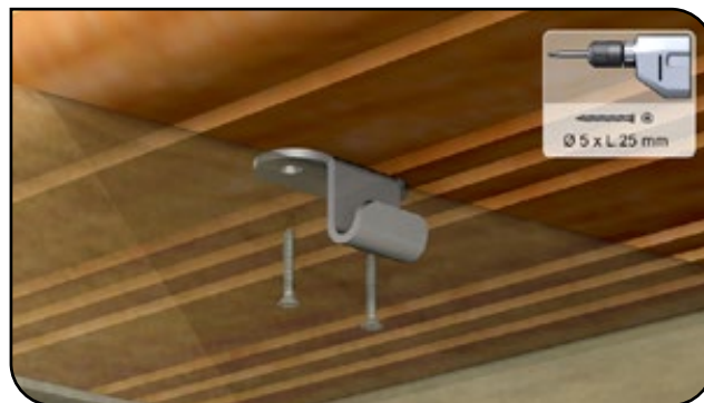
Figure 63 – Crochet sous la margelle
