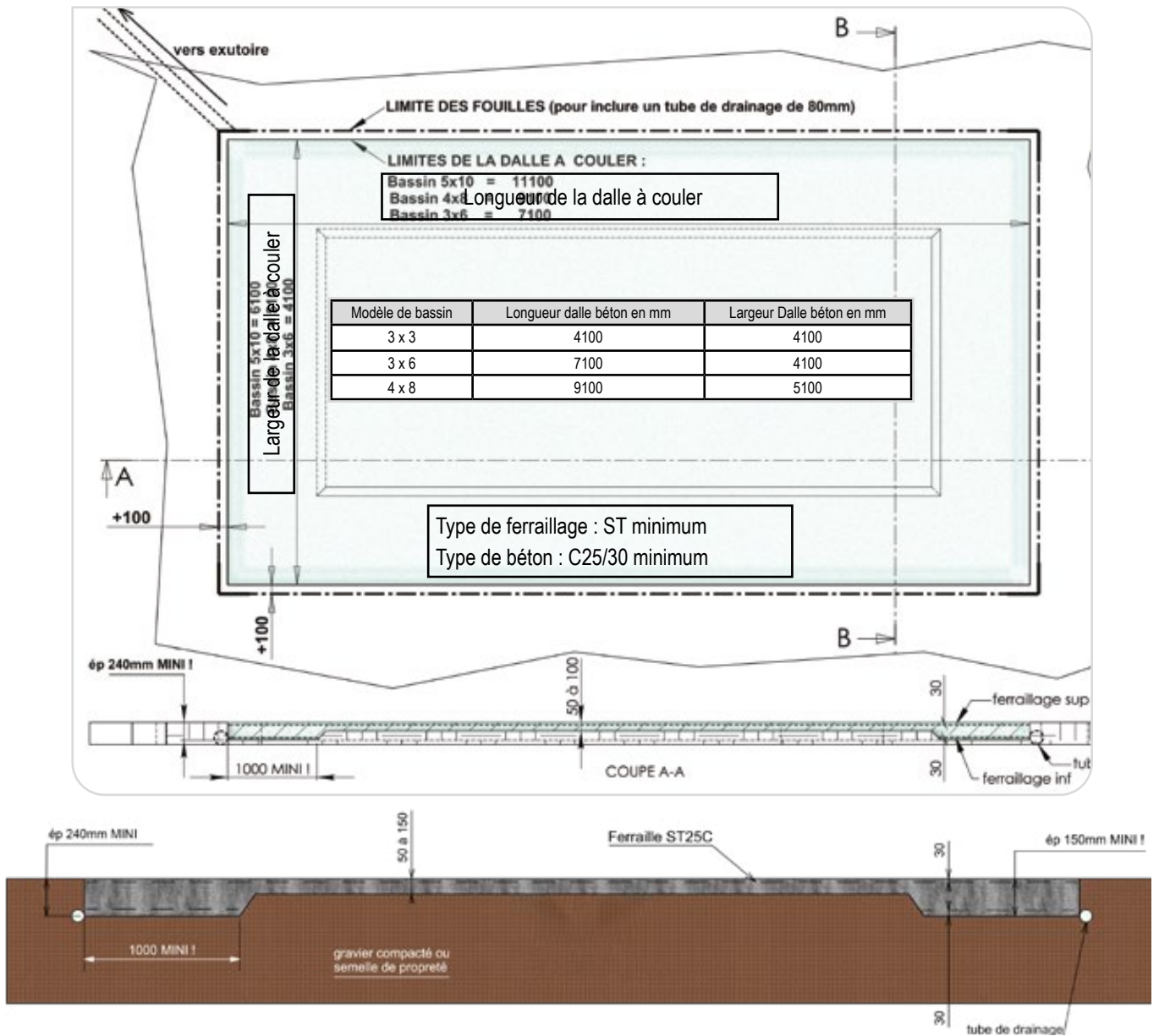
Figure 1 – limites des fouilles et dimensions de la dalle
