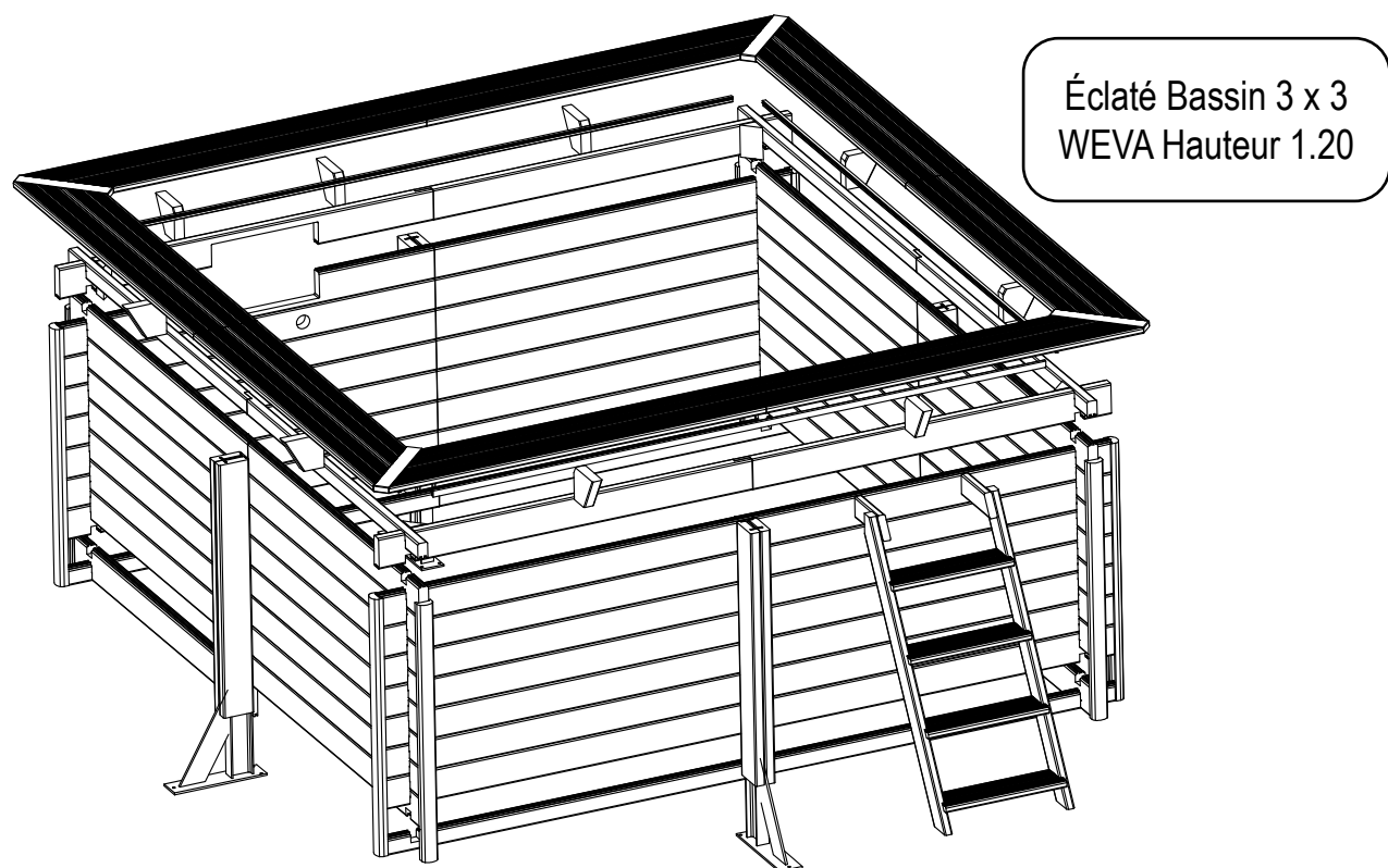
Figure 66 – éclaté bassin 3 x 3 - WEVA Hauteur 1.20
