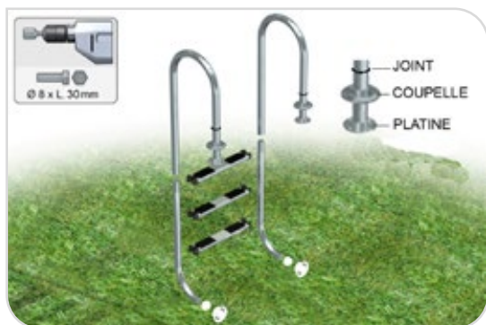
Figure 60 – les parties de l'échelle
