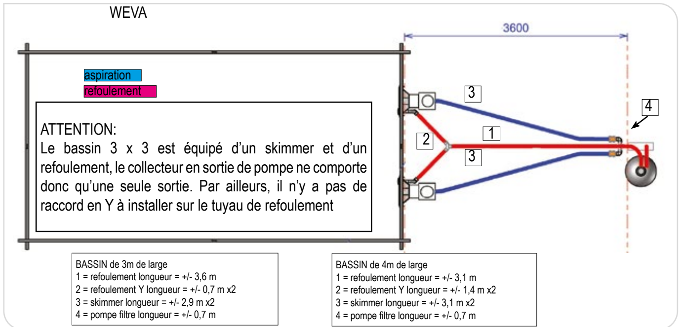
Figure 47 – Exemple de filtration avec deux skimmers - Weva
