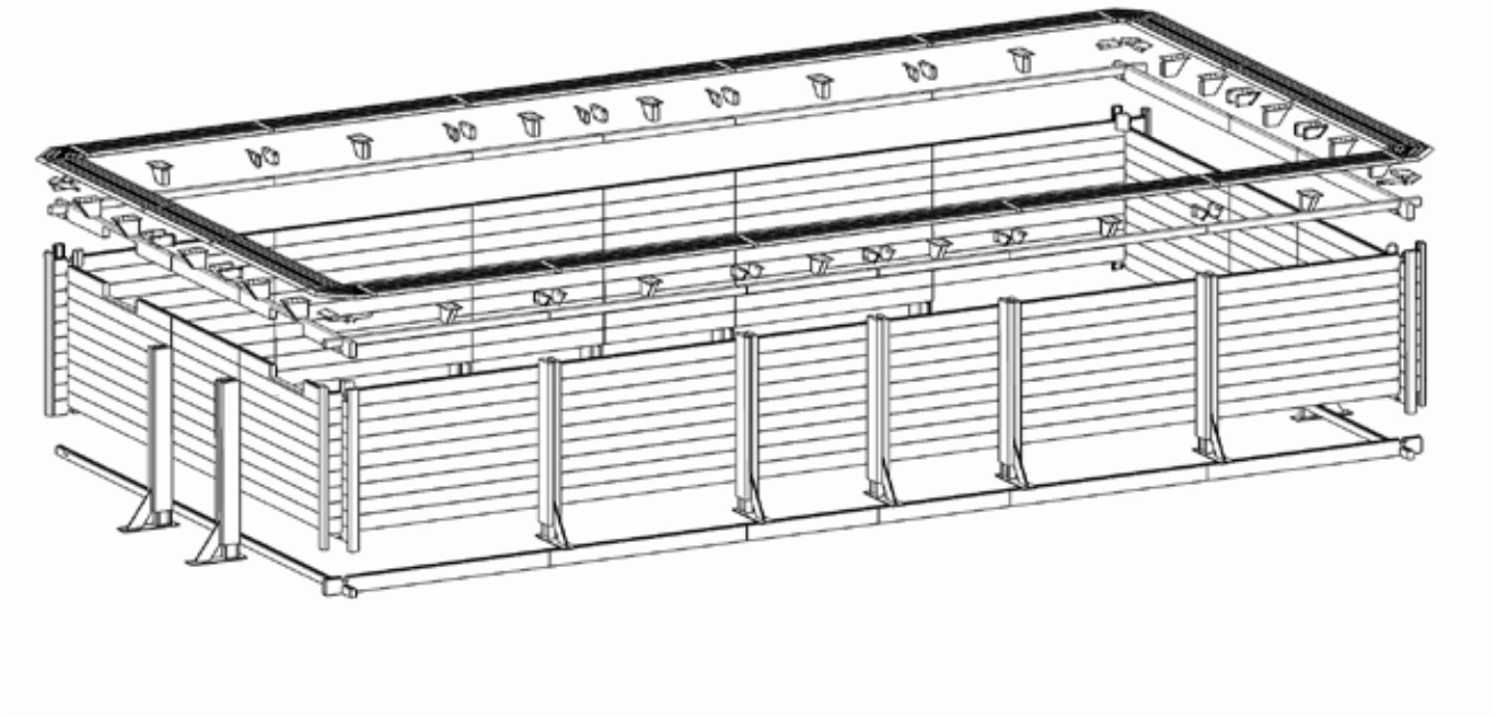
Figure 68 – éclaté bassin 8 x 4 - ODYS SEA Hauteur 1.46
